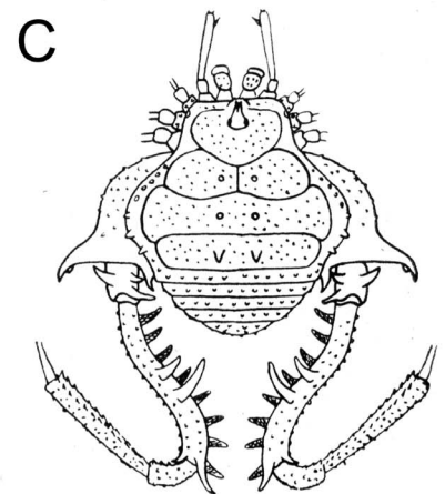
Fig. 610. Gonyleptes curvipes ♂. Körper dorsal mit 4. Bein bis zur Tibia. (Nach Typ.)
