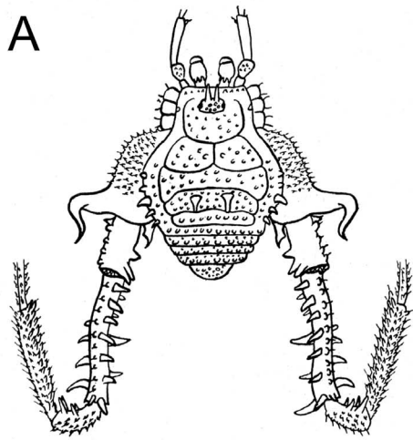
Fig. 544. Discocyrtus curvipes ♂. Körper dorsal mit 4. Bein bis zur Tibia.
