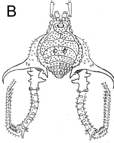
Fig. 546. Discocyrtus crenulatus ♂. Körper dorsal mit 4. Bein bis zur Tibia.
